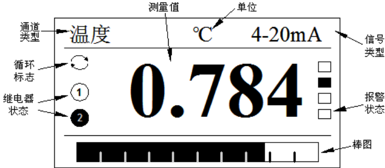
图12 数显画面
