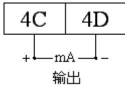
图 7 输出信号接线图
