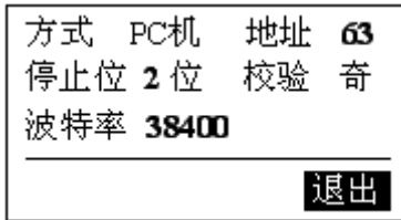
图 33 通讯组态 1
