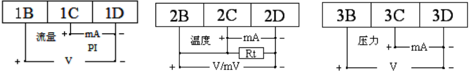
图 4 输入信号（流量、温度、压力）接线图
