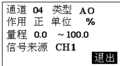
图 36 输出组态画面
