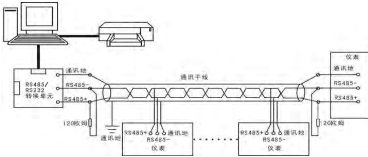
图 40 RS-485 通讯接线方法
