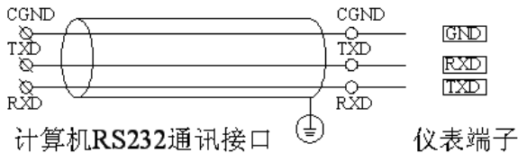
图 39 RS-232 通讯接线方法
