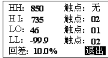
图 32 报警设置
