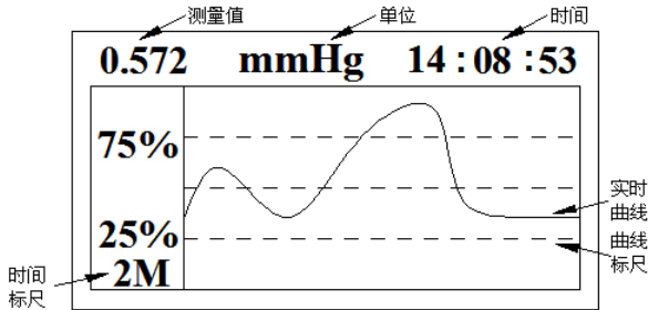
图13 实时曲线
