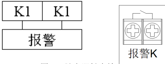
图 5 继电器触点输出接线图
