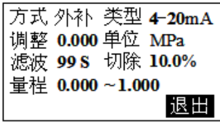
图 28 压力组态 1
