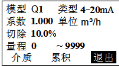
图 24 流量组态
