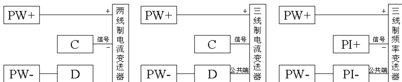
图 6 变送器电源输出接线图
