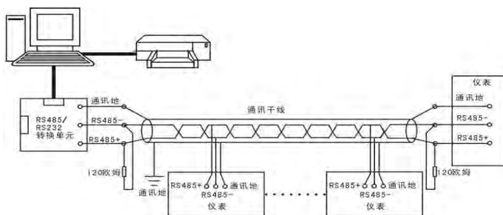
图 27 RS-485 通讯接线方法
