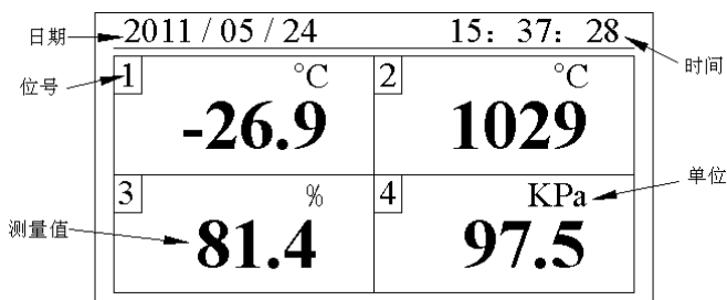
图10 总貌画面
