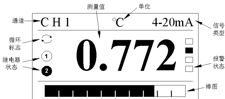
图11 数显画面
