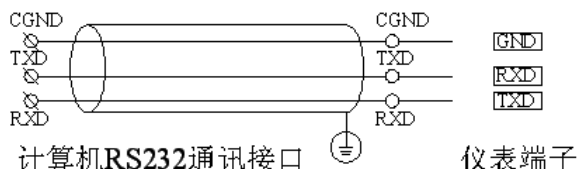
图 26 RS-232 通讯接线方法
