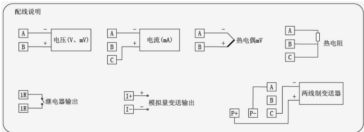
接线图:
