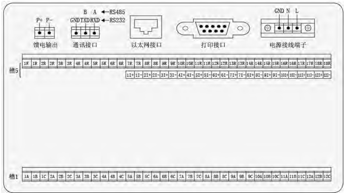
接线图:
