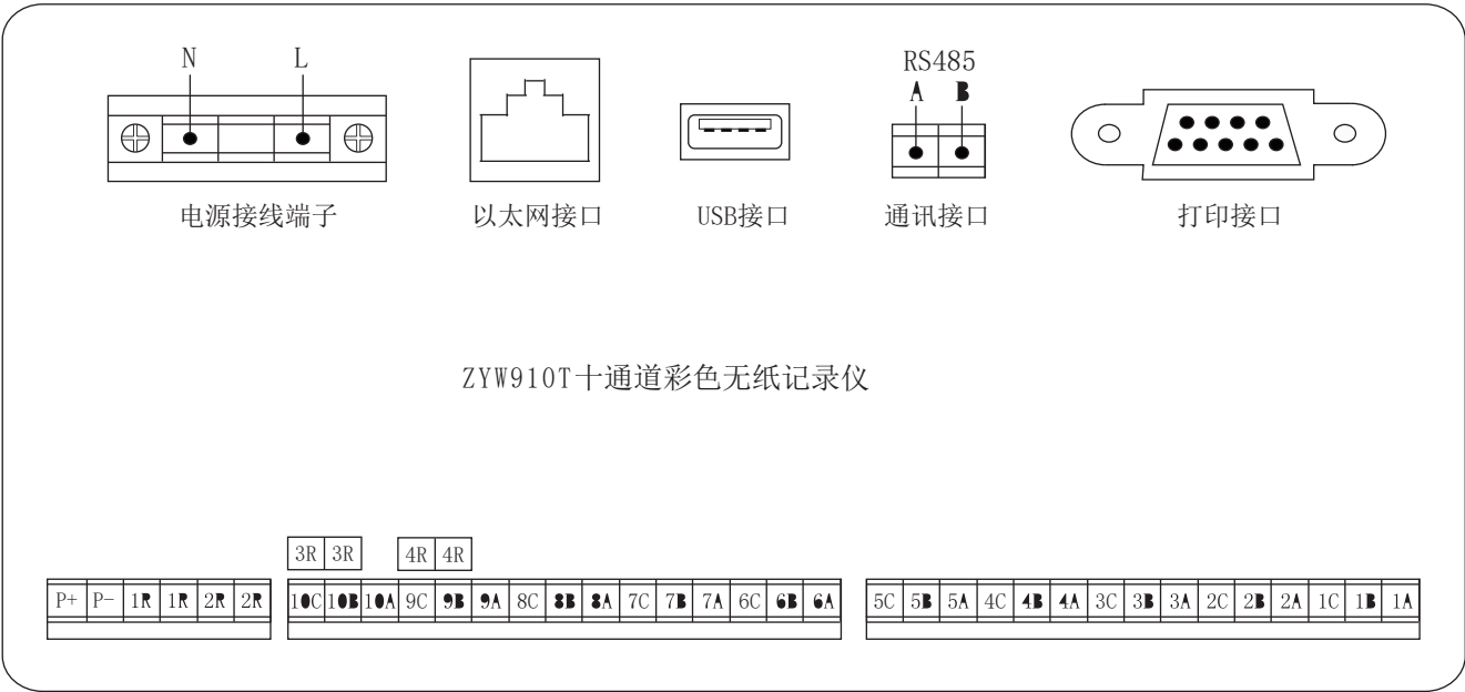
仪表尾部端子图
