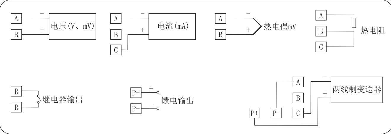
配线说明
